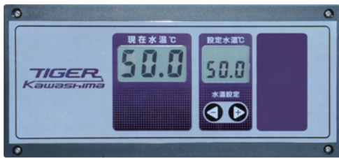
● 制御パネル
